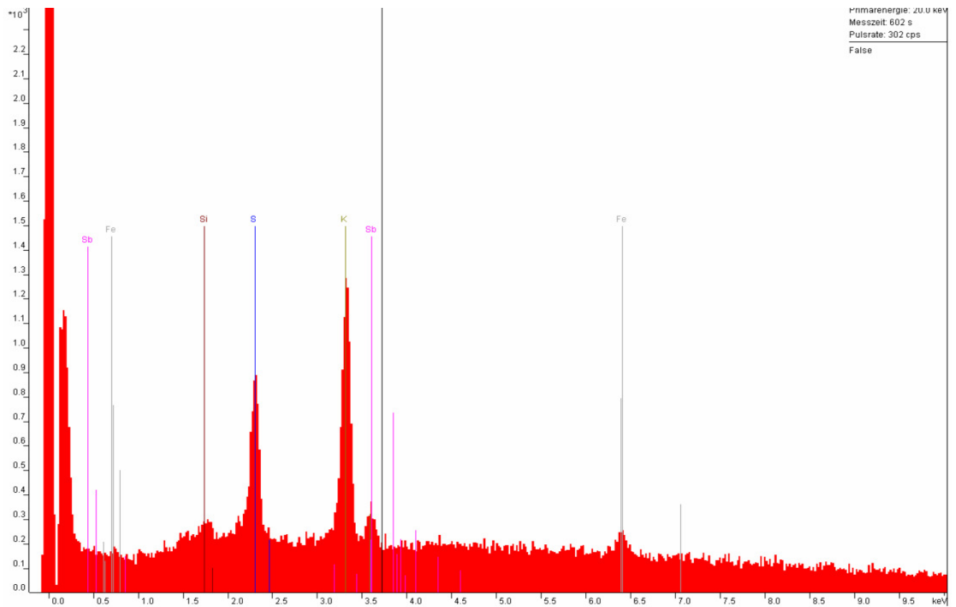
Abb.15, S.21 REM Ergebnisse von der Mumienhaut von Miriam Meyer
