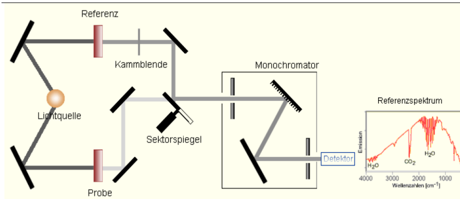
Abb.6, S.10 schematische Darstellung eines IR- Spektrometers
