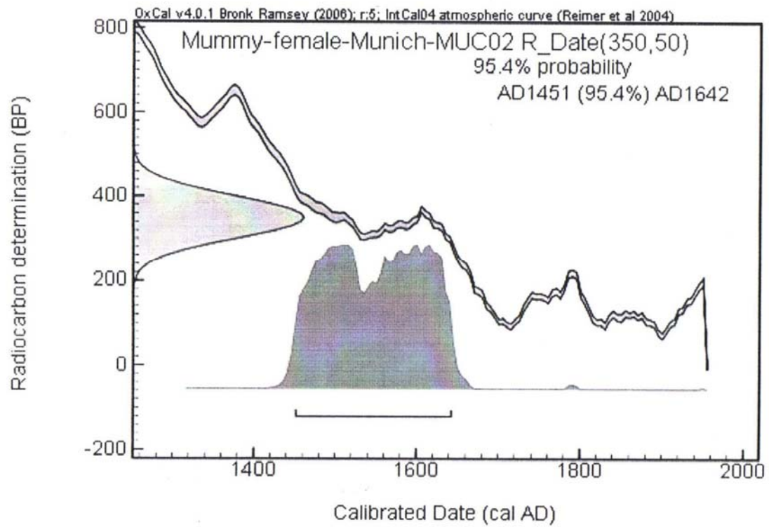
Abb.3, S.7 Auswertung der Radiokarbonmethode: Archäologische Staatssammlung, B. Haas-Gebhard
