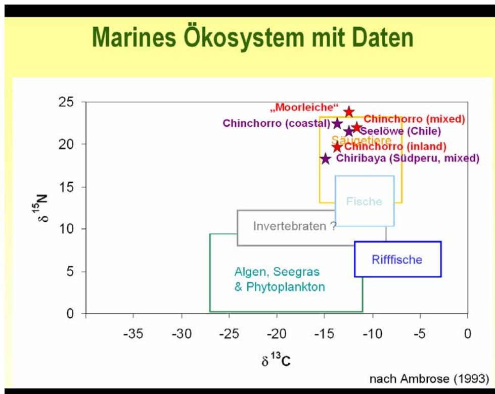
Abb.12, S.18 Marines Ökosystem mit Daten
