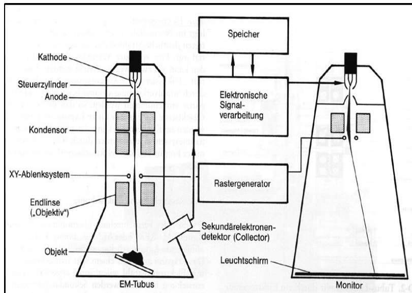
Abb.5, S.8 REM- Apparatur
