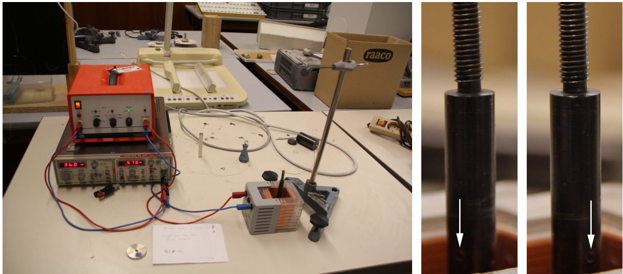
Abb. 3: Links: Übersicht Einstein-de-Haas-Experiment (Links unten: Sinusgenerator; darüber: Verstärker; rechts: Spule mit hineingehängtem Metallstab) Rechts: Beobachtete Maximalausschläge des Stabes; Der Pfeil zeigt jeweils auf die gleiche Stelle des Stabes
