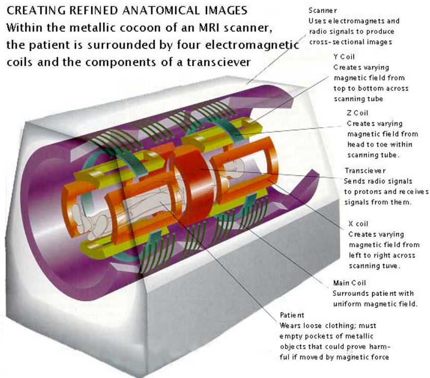
Abb. 5: Der Aufbau eines MRT-Geräts.
