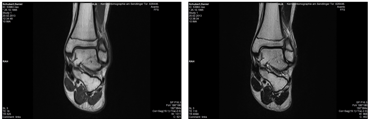
Abb. 12: Das gleiche Bild eines Fußes, links T_1 -gewichtet, rechts T_2 -gewichtet. Rechts erscheinen Flüssigkeiten, die eine lange T_2 haben, hell
