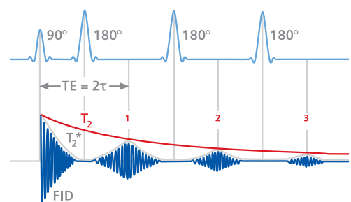
Abb. 8: Die Spinechos fallen mit T2 ab
