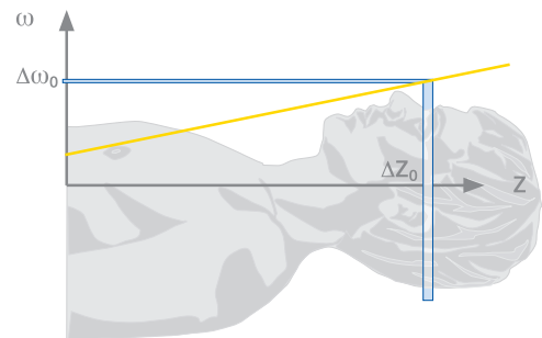
Abb. 9: Die Schichtdicke hängt von der Bandbreite des HF-Pulses und der Steilheit des Gradienten ab
