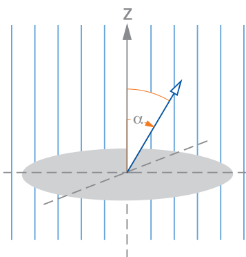
Abb. 6: Die Spins lassen sich entgegen dem Magnetfeld auslenken
