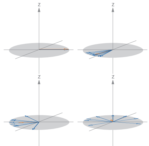
Abb. 7: Mit der Zeit dephasieren die Spins (blau), da einzelne schneller präzedieren, als andere: Die Quermagnetisierung (orange) nimmt ab.
