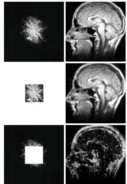
Abb. 13: Aus dem K-Raum wird das Bild generiert.
