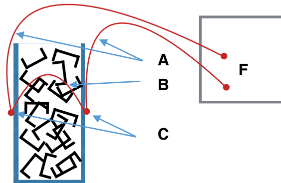
Abb.4: Spannungsmessung am Probekörper
