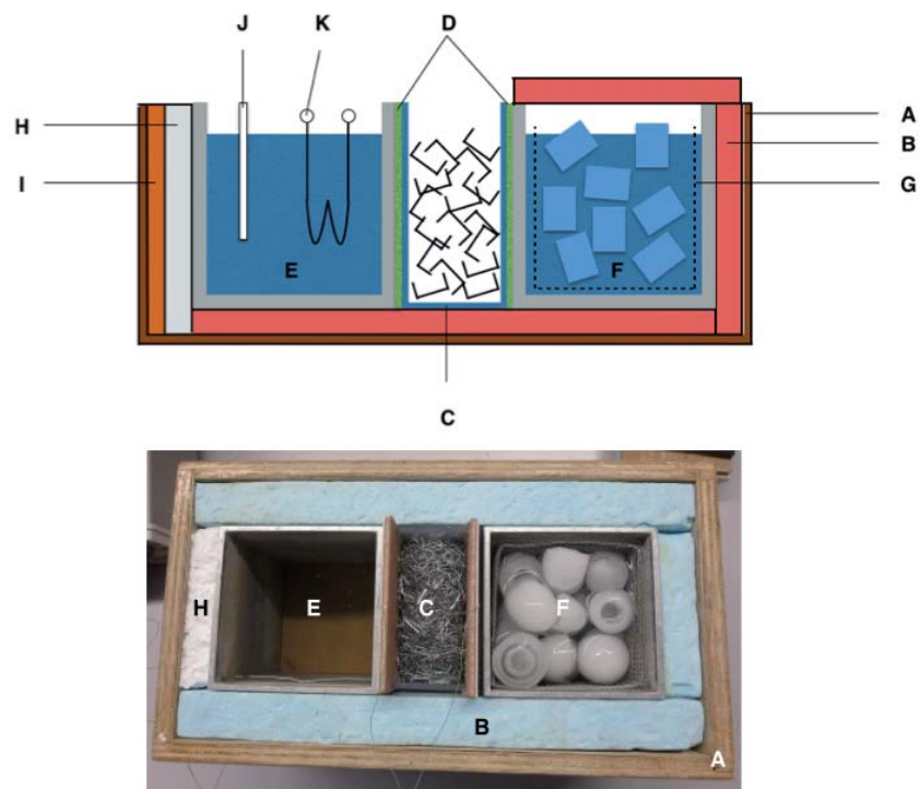
Abb.5: Versuchsaufbau schematisch (oben; modifiziert nach Referenz 7 ) und fotografisch (unten)
